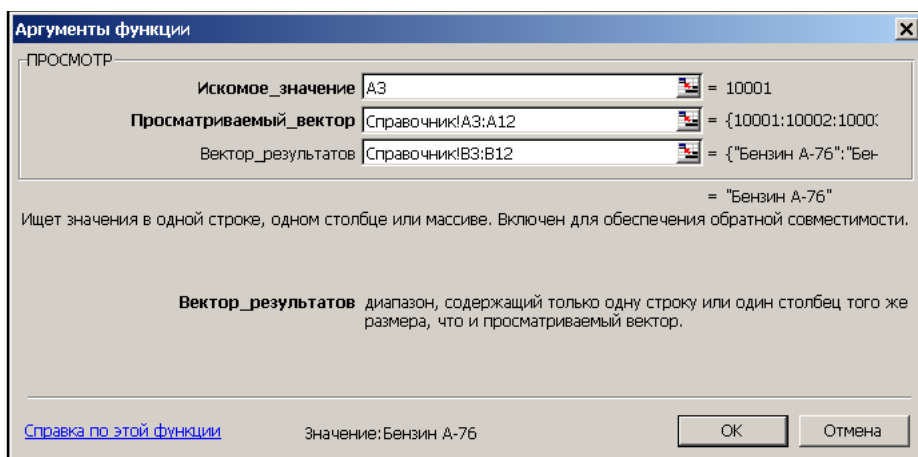
Рис. 236. Заполнение поля «Вектор результатов»
