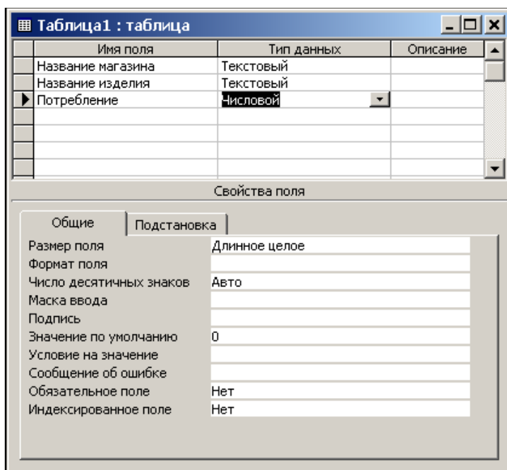
Рис. 60. Ввод структуры таблицы ПОТРЕБЛЕНИЕ
