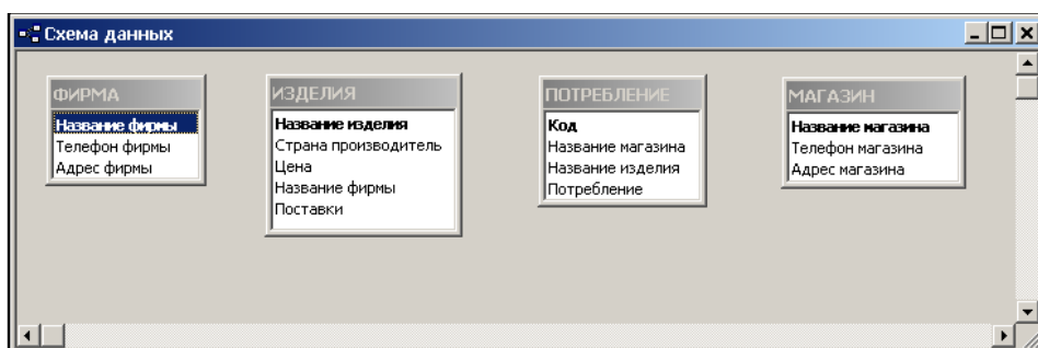
Рис. 65. Окно схемы данных
