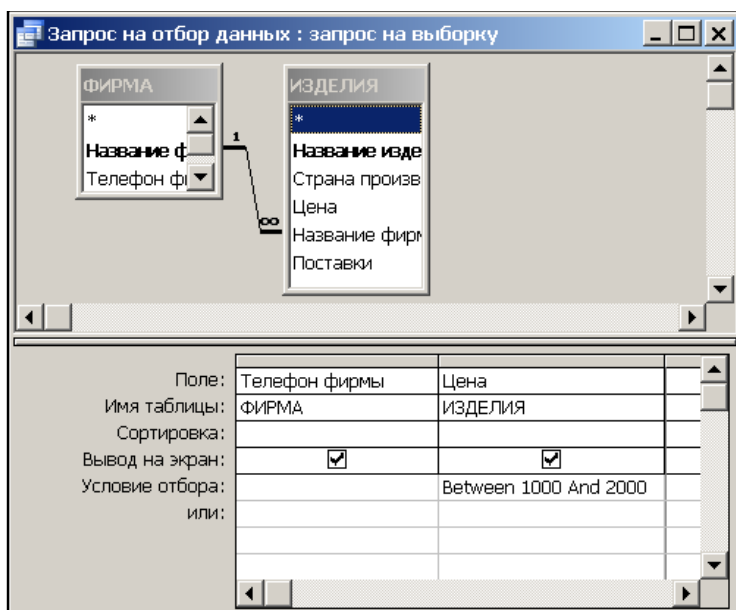
Рис. 92. Создание запроса на отбор данных
