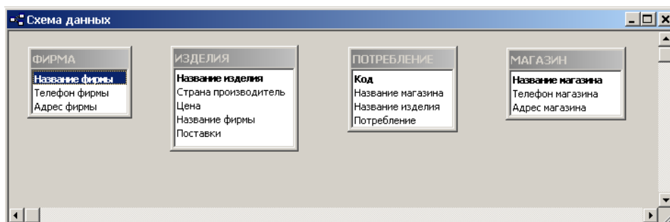
Рис. 85. Окно схемы данных
