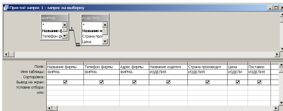
Рис. 91. Форма создания запроса
