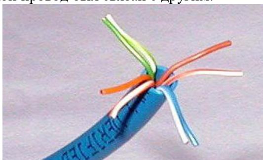
Рис. 4. Расплетение жил
