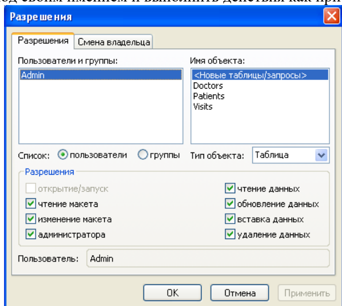
Рисунок 8 - Окно определения прав доступа для каждого пользователя
