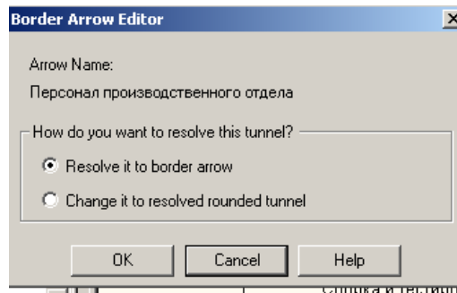
Рисунок 24. Диалог BorderArrowEditor
