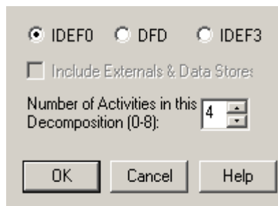
Рисунок 8. Диалог ActivityBoxCount
