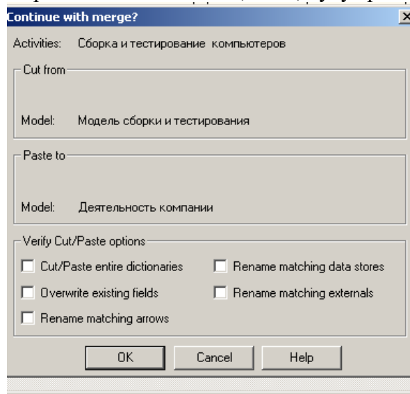
Рисунок 34. Диалог Continewithmerge
