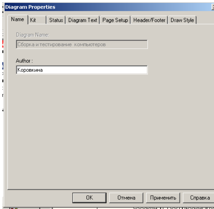
Рисунок 32. Диалог DiagramProperties
