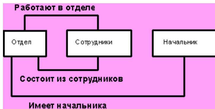
Рис. 6. Пример сетевой схемы БД
