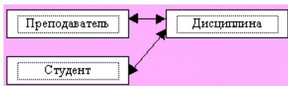
Рис.2. Исходная ER-модель
